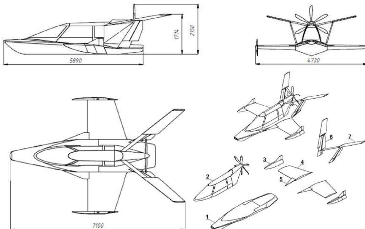
Рис. 1. Предварительная (базовая) аэродинамическая схема экраноплана - трансформера ЭТ-2. 1 - водоизмещающая лодка; 2 - надстройка – кабина с силовой энергетической установкой; 3 - концевые шайбы крыла; 4 - крылья; 5 - подкрылки; 6 - вертикальное оперение (кили); 7 - горизонтальное оперение
