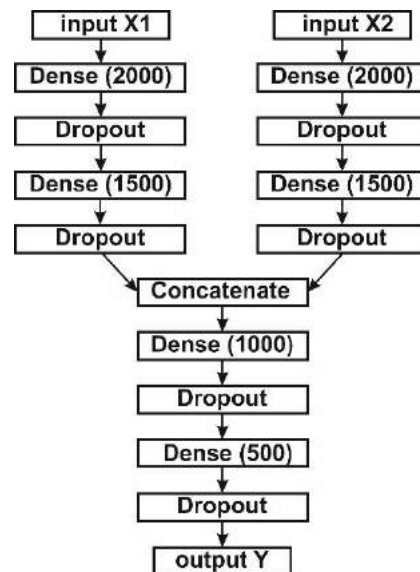
Рис. 3. Нейронная сеть (модель B)
