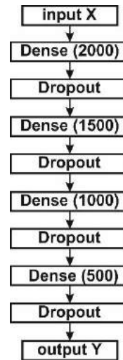
Рис. 2. Нейронная сеть (модель A)
