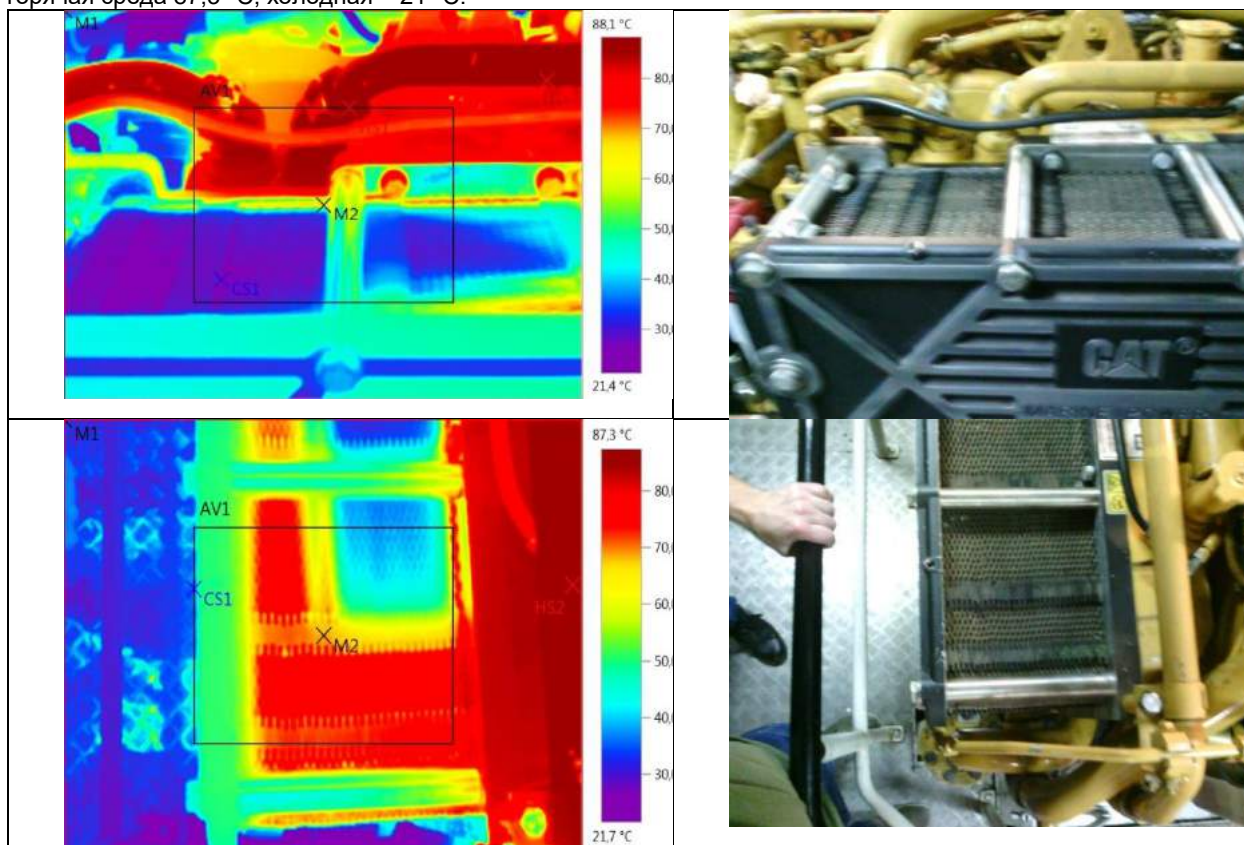
Рис. 6. Термограммы водоводяного охладителя ВОД фирмы "Caterpillar" C32 при нагрузке 66 % от N_{e,ном} во время теплотехнических испытаний а) распределение холодной среды в теплообменнике б) распределение горячей среды в теплообменнике
