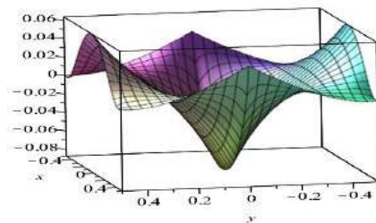
Рис. 5. Изгибающие моменты M_y квадратной пластины. Нагрузка распределена по всей оси Ox пластины ( u=\gamma ).
