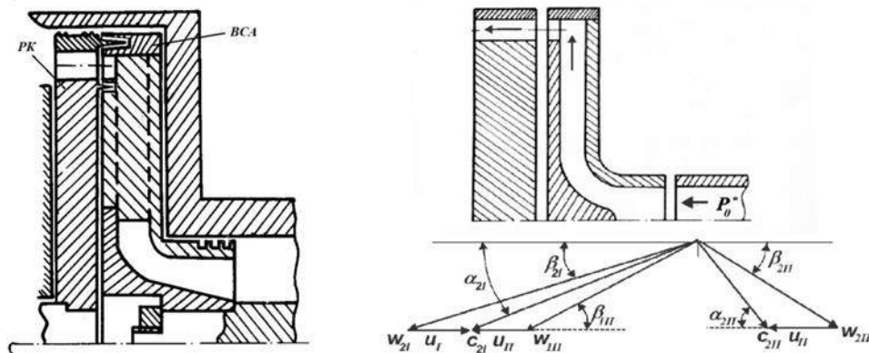
Рис. 3. Биротативная турбина
