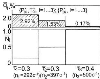
Рис. 3. Сравнение эффективности различных программ регулирования при многорежимной оптимизации МРТ
