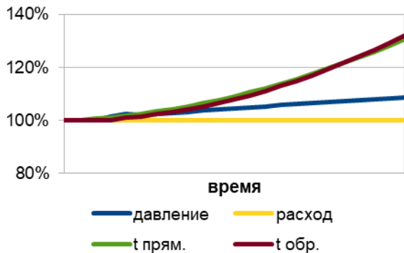
Рис. 2. Показатели работы системы при отключении регулятора
