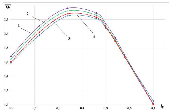
Рис. 11 Зависимость несущей способности от параметра \bar{l}_p при различных значениях \bar{L}_{var} : 1 – \bar{L}_{var} = 0,5 ; 2 – \bar{L}_{var} = 0,3 ; 3 – \bar{L}_{var} = 0,8 ; 4 – \bar{L}_{var} = 0,1 .
