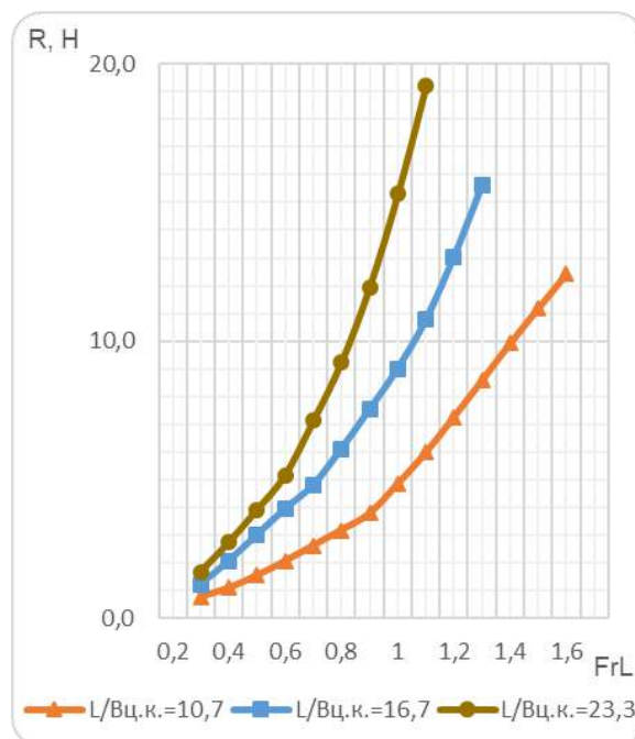
Рис. 5. Сопротивление модели судна-тримарана при носовом расположении аутригеров
