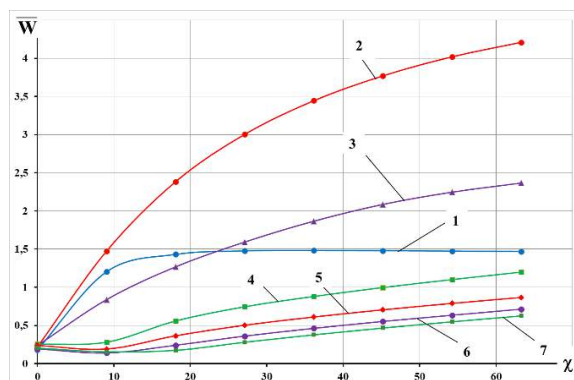
Рис. 10 Зависимость коэффициента несущей способности от числа \chi при различных значениях \psi : 1- \psi=0 ; 2- \psi=1 ; 3- \psi=2 ; 4- \psi=3 ; 5- \psi=4 ; 6- \psi=5 ; 7- \psi=6 .
