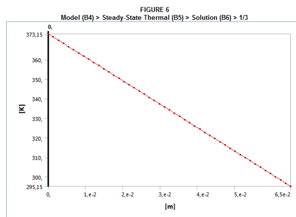
Рис. 6. Распределение температуры по толщине образца
