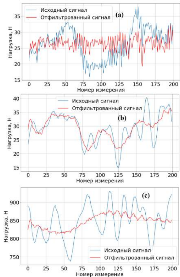
Рис. 7. Графики фрагментов исходных и отфильтрованных продольных нагрузок моделированного льда при пробеге: (а) индентора \varnothing 30 мм, (b) фрагмент модели шириной 700 мм наклонной плоскостью вперед; (с) этой же модели вертикальной плоскостью вперед.
