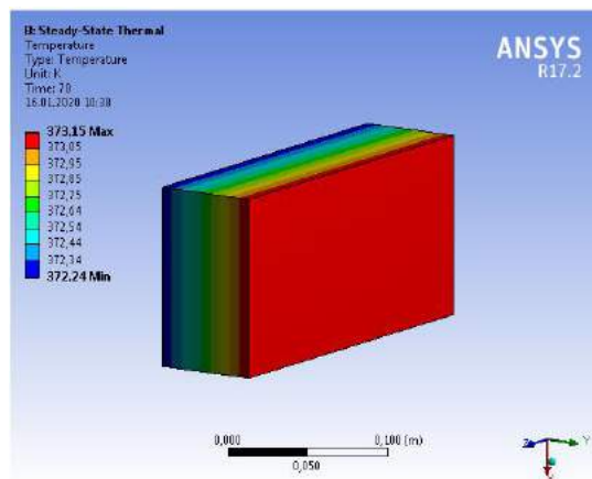
Рис. 4. Температурное поле модели
