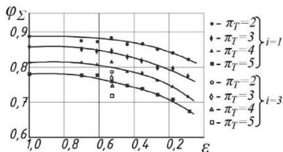
Рис. 3. Коэффициент скорости соплового аппарата при различных значениях \varepsilon и \pi_T
