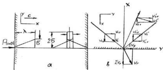
Рис.2. Интерференция акустических волн в металле втулки: c – скорость движения импульса, \lambda – длина волны импульса, \sigma – максимальное напряжение импульса, V_i – скорость падающей волны, V_r – скорость поперечной волны, V_r – скорость проходящей, продольной волны
