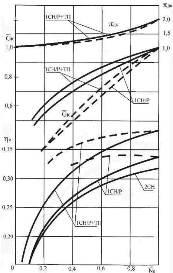
Рис. 3. Характеристик циклов ЗГТУ на частичных винтовых нагрузках при T_3=1373 К, \pi_k=5-6 , \pi_{дж}=2,0 и \sigma=0,8
