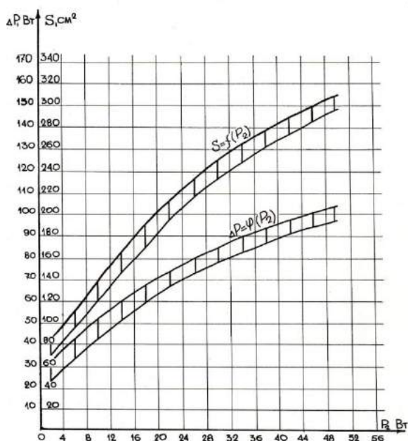
Рис. 1. Зависимость наружной поверхности и потерь от полезной мощности.
