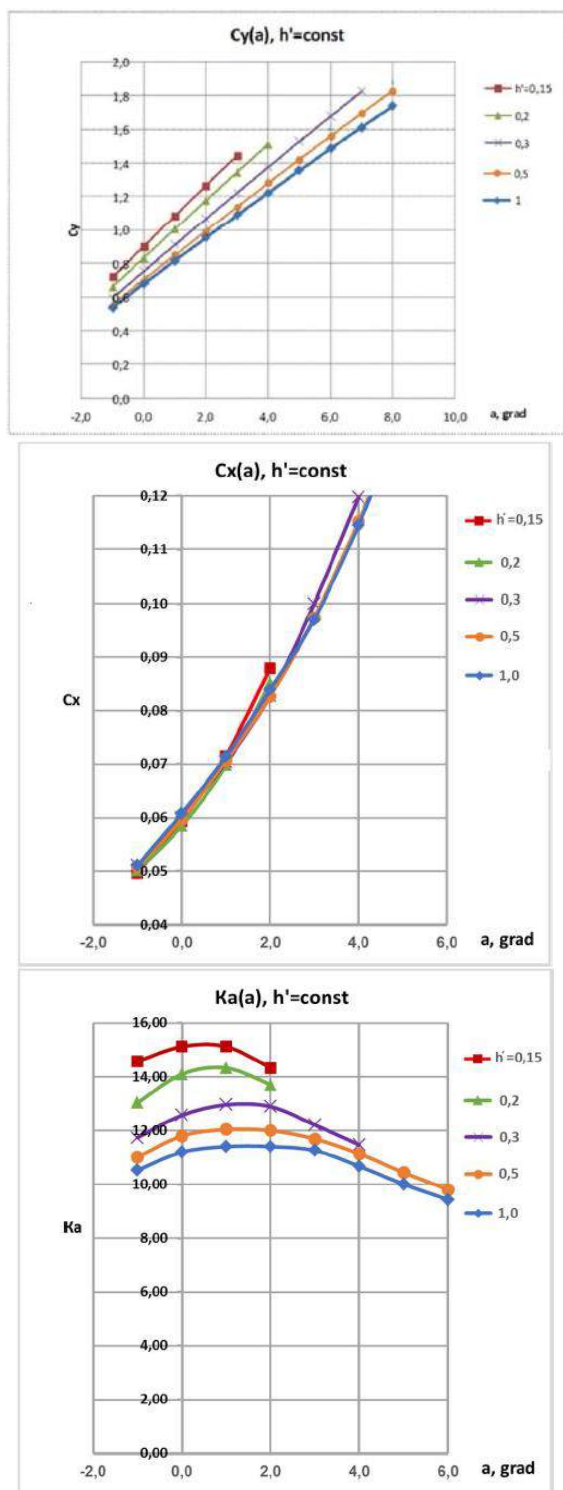
Рис. 7. Аэродинамические характеристики базовой модели экраноплана - трансформера ЭТ-2 C_y=f(\alpha^\circ, h') , C_x=f(\alpha^\circ, h') , K_a=f(\alpha^\circ, h')
