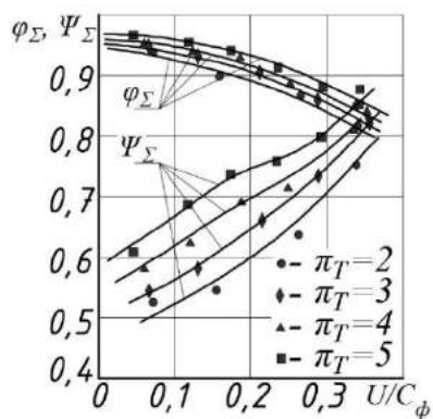
Рис. 1. Коэффициенты скорости СА и РК при различных режимах работы ступени
