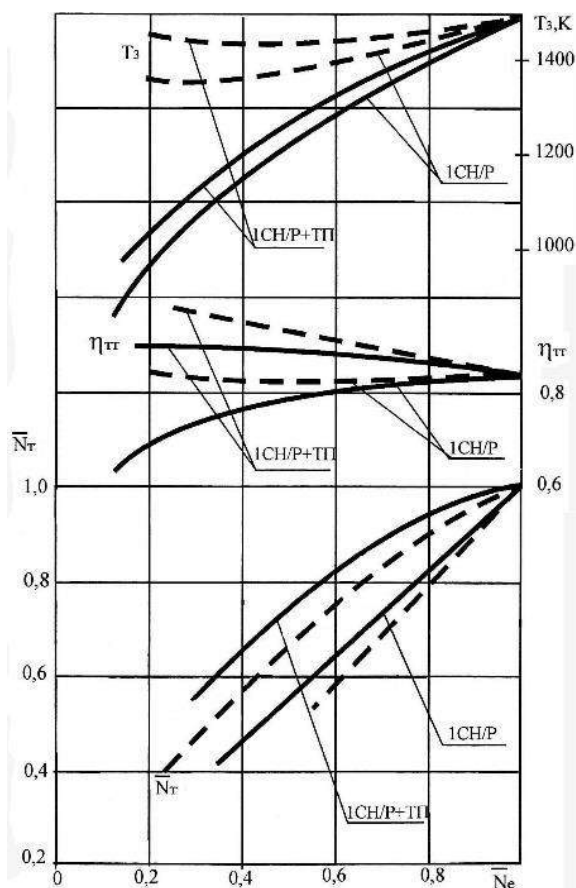
Рис. 4. Теплотехнические характеристики ЗГТУ на частичных винтовых нагрузках при T_3=1373 К, \pi_k=5-6 , \pi_{дж}=2,0 и \sigma=0,8
