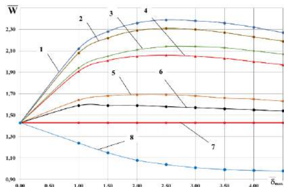
Рис.7 Зависимость коэффициента несущей способности от \bar{\delta}_{max} при различных значениях \bar{L}_{var} : 1 - \bar{L}_{var} = 0,4 2 - \bar{L}_{var} = 0,3 ; 3- \bar{L}_{var} = 0,5 ; 4 - \bar{L}_{var} = 0,2 ; 5 - \bar{L}_{var} = 0,1 ; 6 - \bar{L}_{var} = 0,6 ; 7 - \bar{L}_{var} = 0 ; 8 - \bar{L}_{var} = 0,7 .
