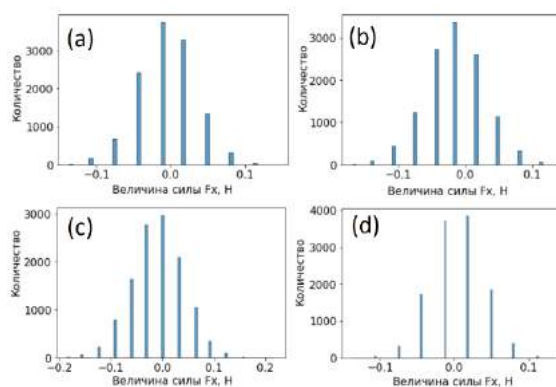
Рис. 4. Гистограммы для данных без всплеска при скоростях: (а) 1 мм/с, (б) 3 мм/с, (с) 5 мм/с, (д) 10 мм/с.
