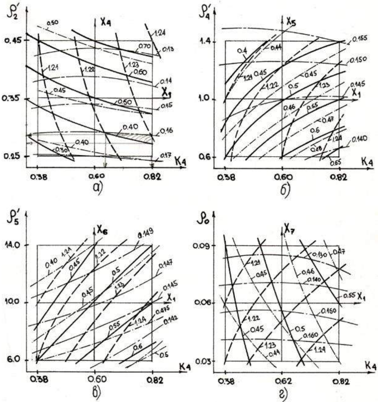
Рис. 2. Номограммы для выбора значений относительных параметров ОАД.
