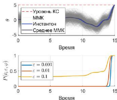
Рис. 4. Траектории, вдоль которых достигается КС крена \theta = 5 при ветре 10 \text{ м/с} в борт.
