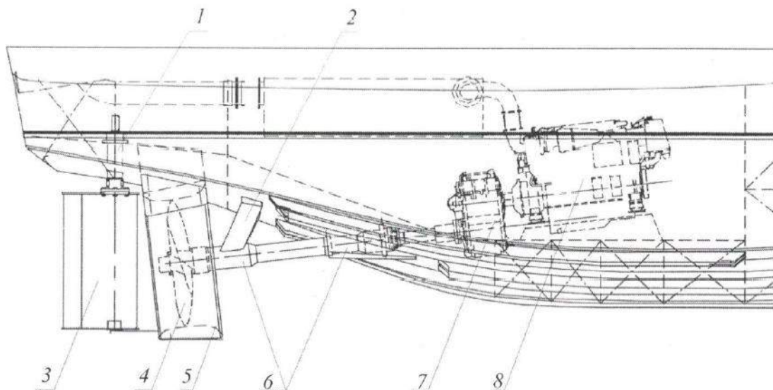
Рис. 1. Пропульсивный комплекс с подвесным дейдвудным устройством проектов 2608 и 1907 Damen stan tug 1 – баллер; 2 – кронштейн валопровода; 3 – перо руля; 4– винт; 5 – насадка; 6 – дейдвудная труба с подшипниками; 7 – редуктор; 8 – главный двигатель
