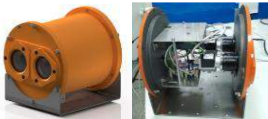
Рис. 1. Действующая подводная система технического стереозрения (а) вид модуля в собранном состоянии (б) внутренняя часть модуля
