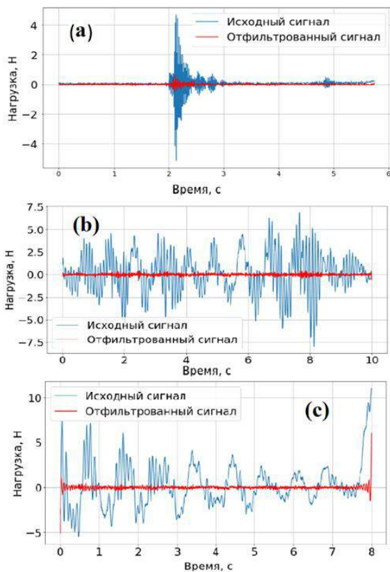
Рис. 6. Графики фрагментов исходных и отфильтрованных показаний канала Fx при пробеге по чистой воде: (а) индентора \varnothing 30 мм, (b) фрагмент модели шириной 700 мм наклонной плоскостью вперед; (с) этой же модели вертикальной плоскостью вперед.
