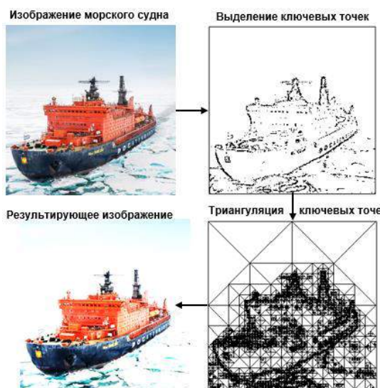
Рис. 3. Процесс сжатия по КТО изображений
