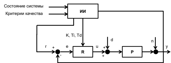
Рис.4. Схема нейросетевого управления
