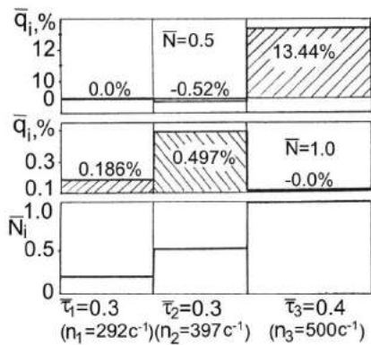
Рис. 1. Увеличение \bar{Q} в ЭУ при оптимизации на i -тые режимы по сравнению с многорежимной для программы регулирования \{P_{0i}^*, T_{0i}^*, Z_{ci}, i = 1 \dots 3\}
