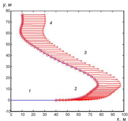
Рис. 8. Перемещение судна лагом по заданной траектории
