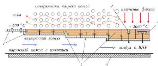
Рис. 1. Схема обмуровки судового котла: 1 – изоляция внутреннего кожуха; 2 – шамотные кирпичи; 3 – высокотемпературное изделие; 4 – мертль; 5 – изоляция наружного кожуха; ВТУ – воздухонаправляющее устройство
