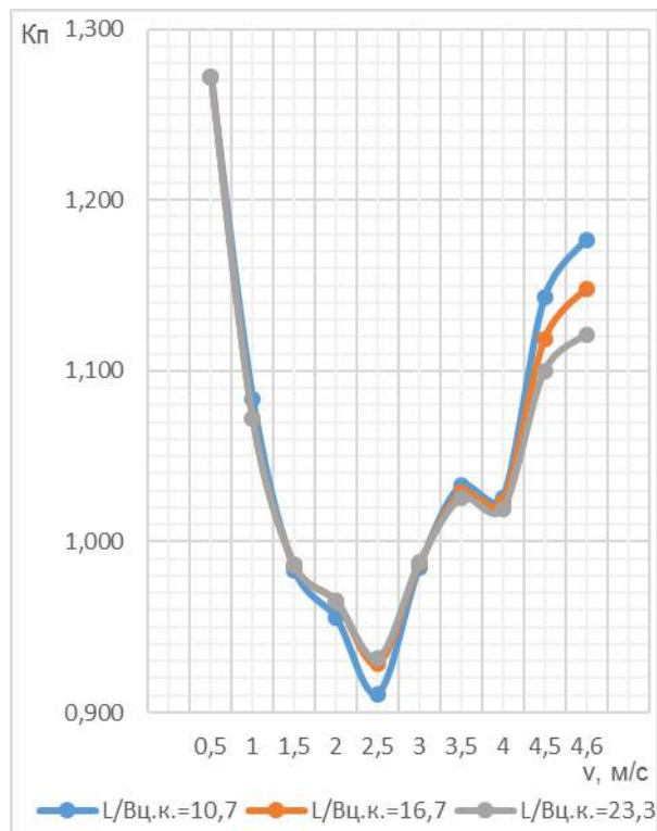
Рис. 9. Поправочный коэффициент при кормовом расположении аутригеров и отношении b/B=0,34
