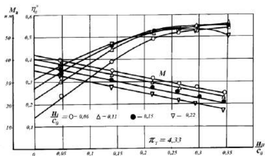
Рис. 4. Изменение внутреннего КПД и крутящего момента биротативной турбины в зависимости от характеристического числа РК при изменении характеристического числа ВСА
