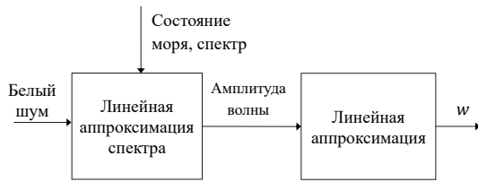
Рис. 2. Схема формирования сил и моментов внешнего возмущения
