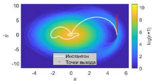
Рис. 5. Плотность траекторий на фазовой плоскости. Сравнение метода Монте-Карло с инстантоном ( \theta = 5^\circ при ветре 10 \text{ м/с} в борт).
