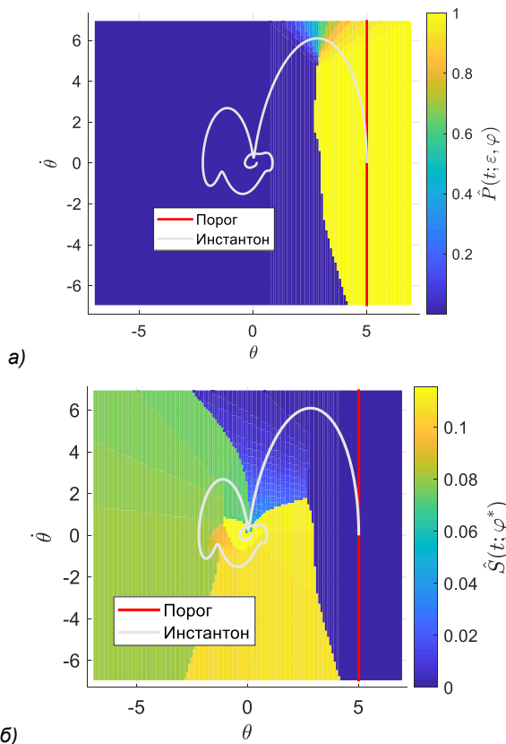
Рис. 10. Оценки вероятностей (а) и квазипотенциалов (б) движения вдоль инстантона к критическому состоянию крена 6 градусов (красная линия). Белой линией указан инстантон.
