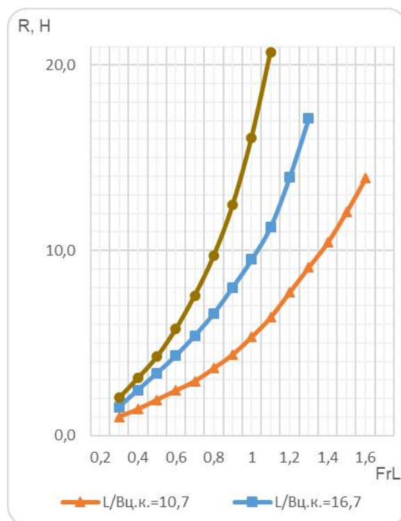
Рис. 6. Сопротивление модели судна-тримарана при центральном расположении аутригеров
