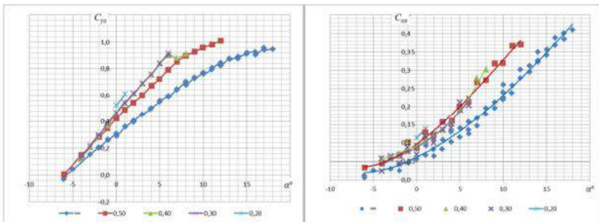
Рис. 4 Результаты измерений коэффициентов подъемной силы, C_p и лобового сопротивления C_x при разных отстояниях h' от экрана в аэродинамической трубе Т3 СГАУ
