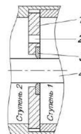
Рис. 4. Уплотнения диафрагмы
