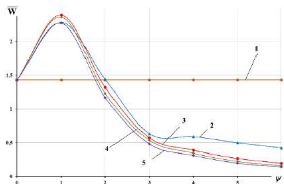
Рис.2 Зависимость коэффициента несущей способности от \psi при различных значениях \bar{\delta}_{max} : 1- \bar{\delta}_{max} = 0 ; 2 - \bar{\delta}_{max} = 1,5 ; 3 - \bar{\delta}_{max} = 2,5 ; 4 - \bar{\delta}_{max} = 4,5 ; 5 - \bar{\delta}_{max} = 4,5
