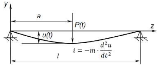
Рис.1. Расчетная схема определения вынужденных колебаний цилиндрической втулки под действием боковой силы от перекадки поршня
