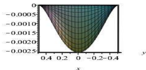
Рис. 2. Прогибы квадратной пластины (вид со стороны оси Oy ). Нагрузка распределена по всей оси Ox пластины ( u=\gamma ). w(0, 0) = -0.0026072
