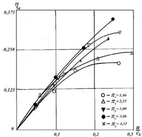
Рис. 2. Характеристики одноступенчатой турбины типа ВСА
