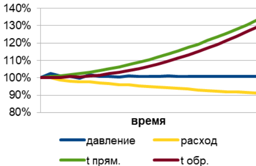
Рис. 3. Показатели работы системы при включении регулятора по давлению
