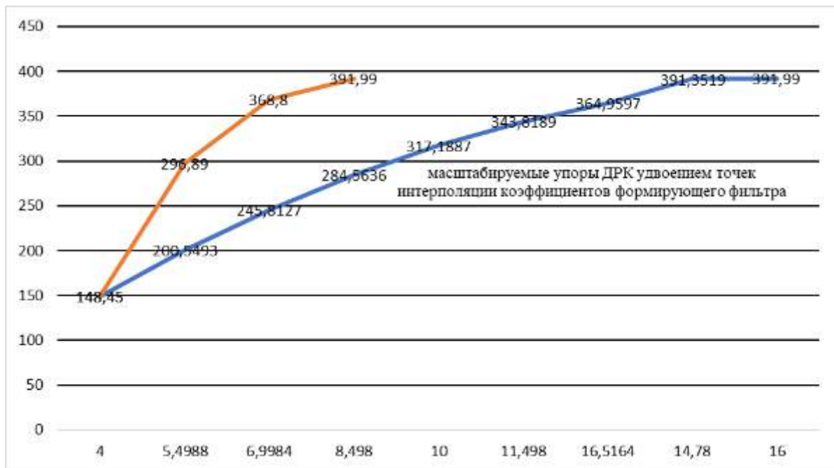
Рис. 5 Масштабирование упоров ДПК удвоением точек интерполяции анализирующего фильтра Добеши с пересчётом к упорам движителей
