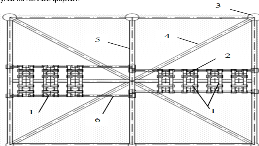
Рис. 3. Раскрепление водоотделяющих колонн с помощью жестких рам (вид в плане на диафрагму МСП):
