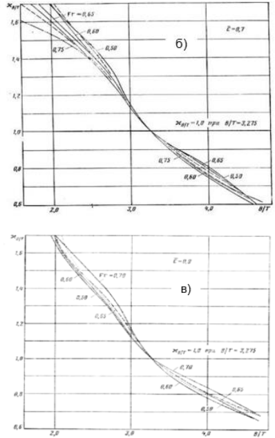
Рис. 4. Графики влияния отношения B/T на изменение остаточного сопротивления катамаранных судов а) для C = 0,5 ; б) для C = 0,7 ; в) для C = 0,9
