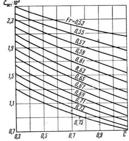
Рис. 5. График влияния клиренса на остаточное сопротивление катамаранных судов
