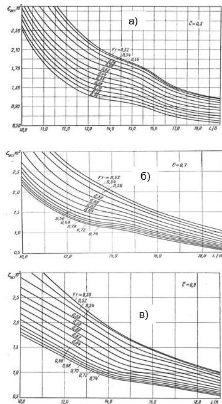
Рис. 2. Диаграмма группы "L/B" для расчета остаточного сопротивления катамаранов \zeta_{ост}^{L/B} а) для \delta = 0,5 б) для \delta = 0,7 в) для \delta = 0,9
