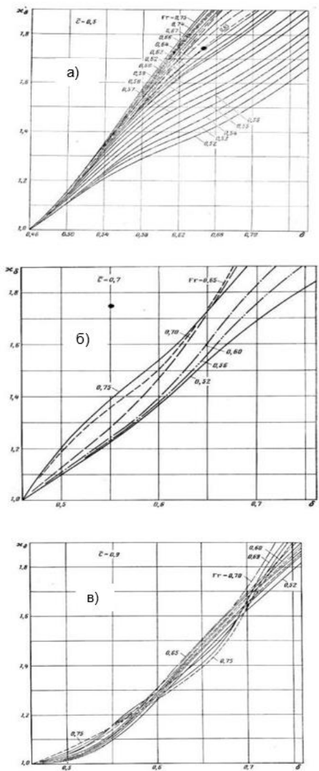
Рис. 3. Графики влияния параметра \delta на изменение остаточного сопротивления катамаранных судов а) для C = 0,5 ; б) для C = 0,7 ; в) для C = 0,9
